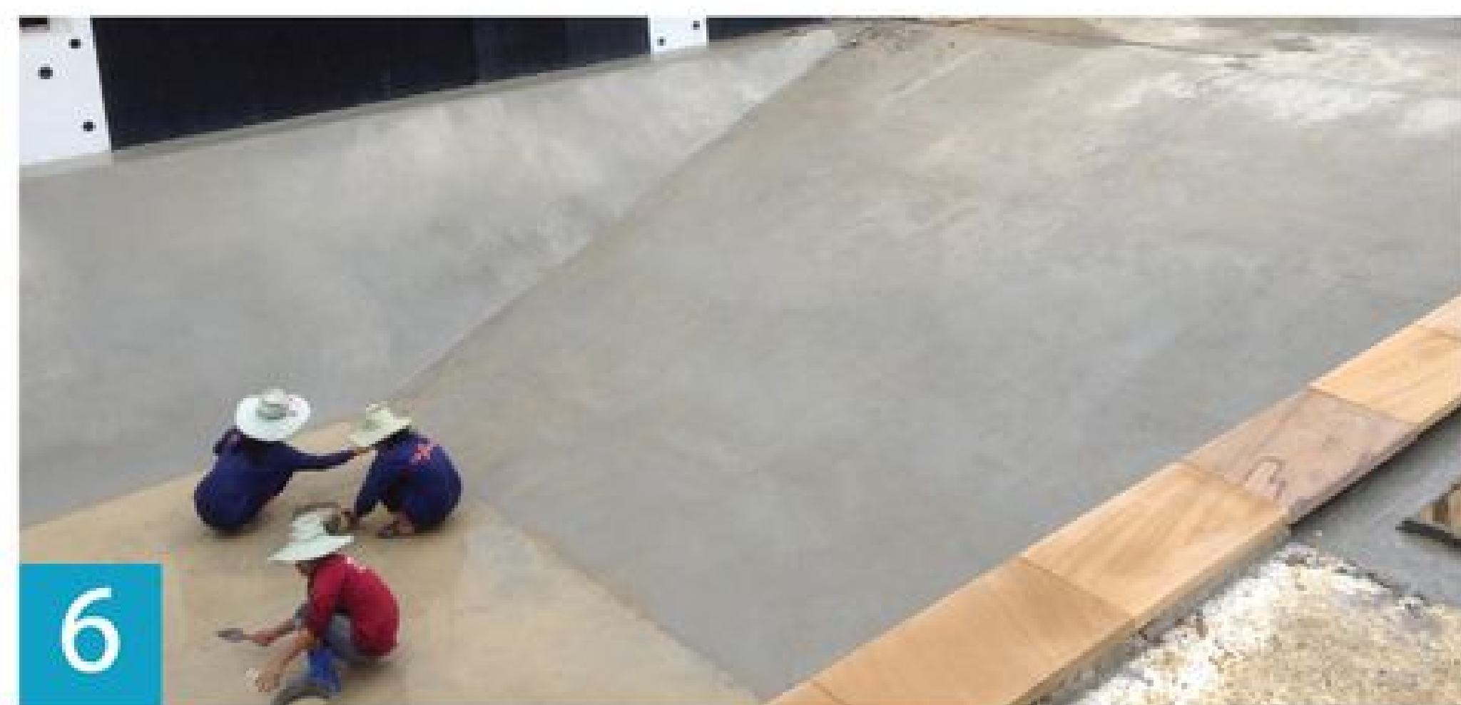
6 Laying coping stones and then ready for PVC lining วางหินทรายขอบสระ และเตรียมงานไลเนอร์
